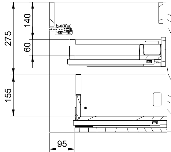
A-A ( 1 : 8 )
